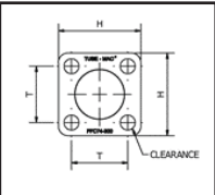
F10 Flare Flange Dimensions NPS Page K1
