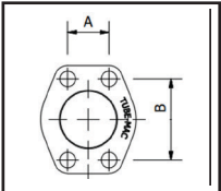
90° Flare Flange Dimensions Page D1
