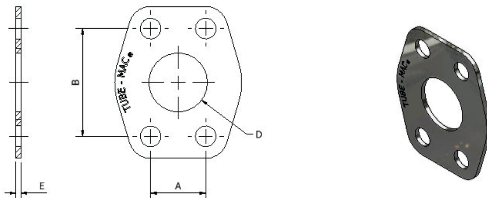
CP - Connector Plate
